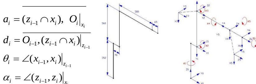
Modelo de Coordenadas Robô ABB IRB140
