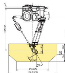
Robô Fanuc M3iA/6. Fonte Fanuc Robotics.
